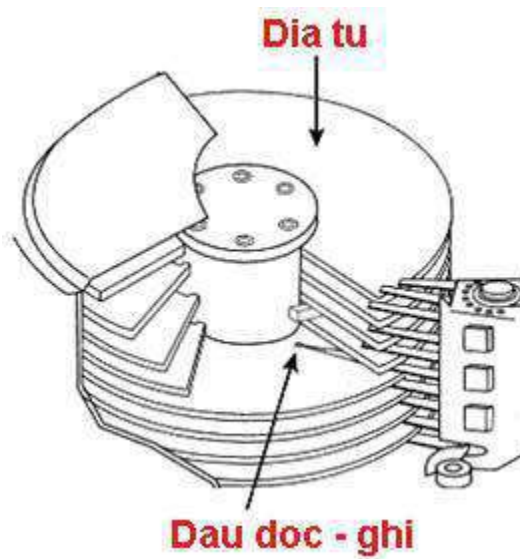
Cấu tạo bên trong ổ cứng
