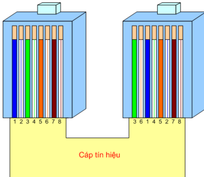
Cáp mạng đầu chéo
