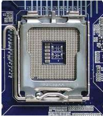
Đế cắm CPU Socket 775
