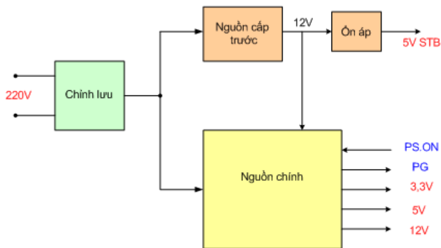
Sơ đồ mạch tổng quát của bộ nguồn ATX
