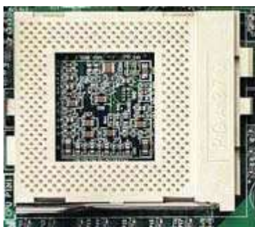
Đế cắm CPU - Socket370 trong các máy Pentium 3
