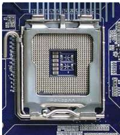
Đế cắm CPU - Socket 775 trong các máy Pentium 4 đời mới
