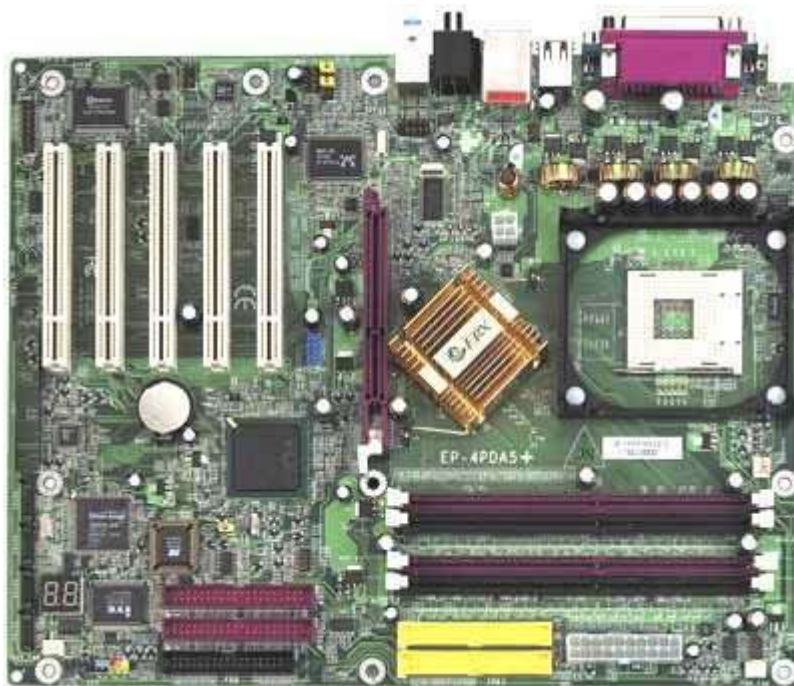
Mainboard máy Pentium 4 ( Đời trung ) - Socket 478
