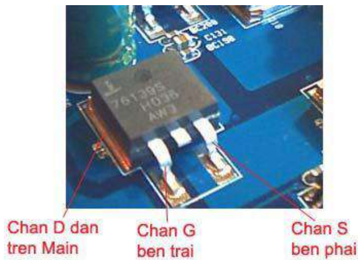
Đèn Mosfet điều khiển nguồn
