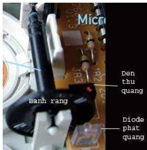
Bộ cảm biến trong chuột bi
