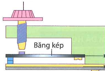
b) Băng kép đóng ngắt mạch điện
