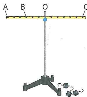
Hình 18.1 Dụng cụ thí nghiệm
