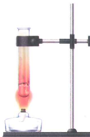
Hình 2.2 Thí nghiệm sắt phản ứng với lưu huỳnh
