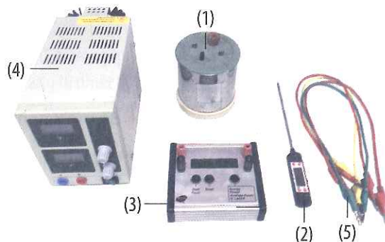
Hình 27.1 Dụng cụ thí nghiệm đo năng lượng nhiệt
