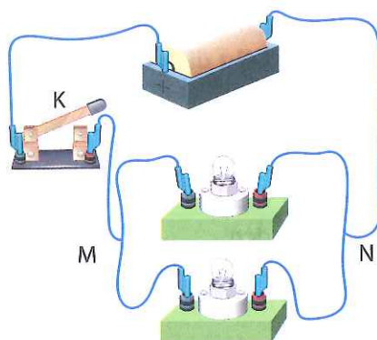
b) Hai bóng đèn mắc song song
