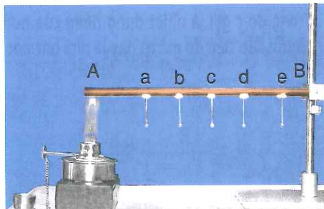
Hình 28.1 Bố trí thí nghiệm tìm hiểu sự dẫn nhiệt
