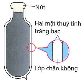
Hình 28.6 Cấu tạo ruột phích (bình thủy)
